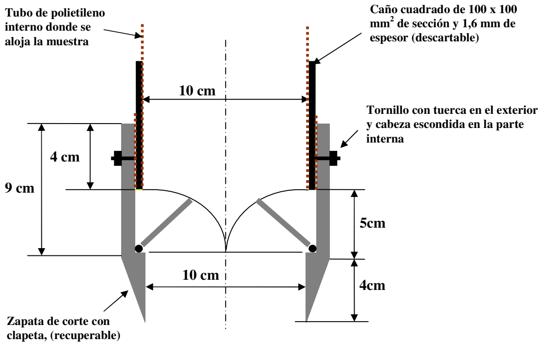
Figura N° 1: Esquema de la zapata de corte de sección cuadrada con clapeta de cierre
